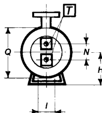
CONFIGURAZIONE - shape COPERTURA TIPO "B" cover type
